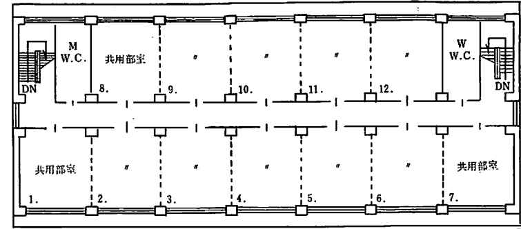
<3階平面図 S:1/300> (注:各室は必要に応じて区切る)
