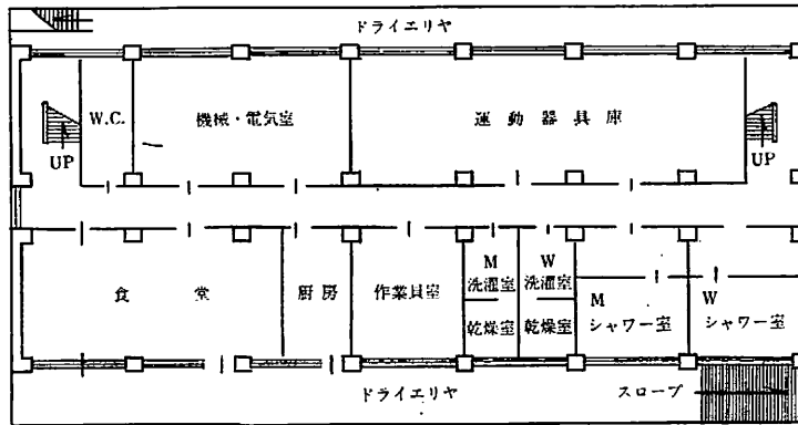
<地階平面図 S:1/300>
