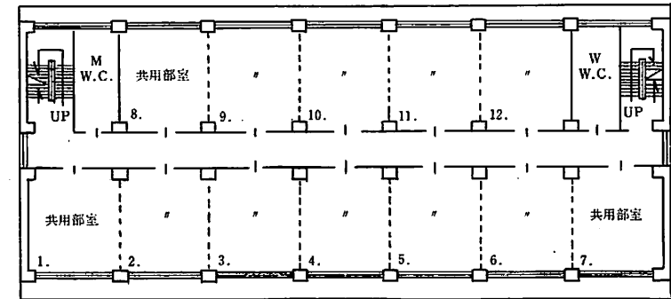
<2階平面図 S:1/300> (注:各室は必要に応じて区切る)
