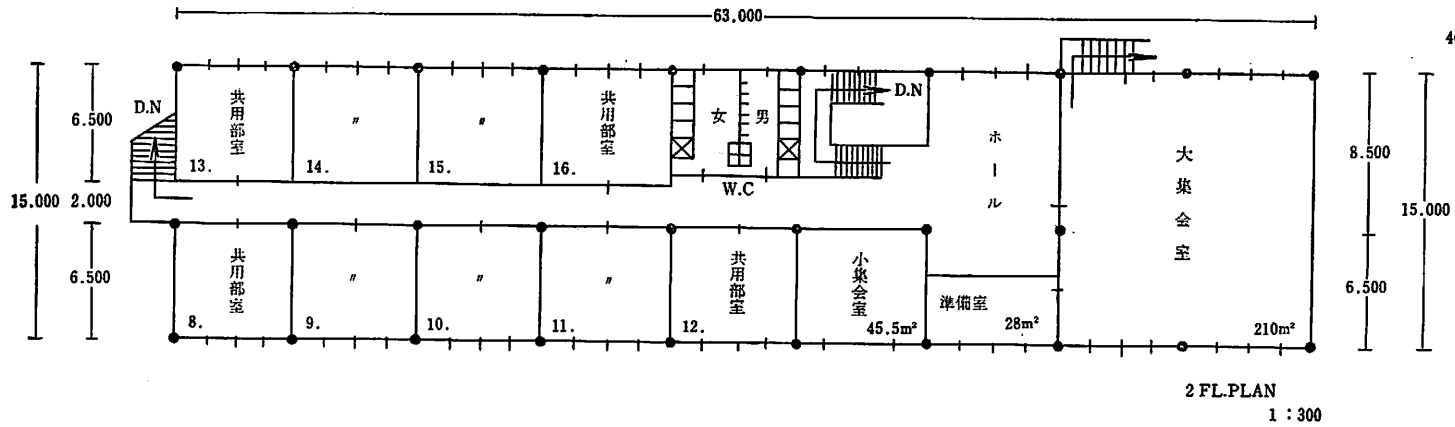
体育サークル会館の平面図(1)
