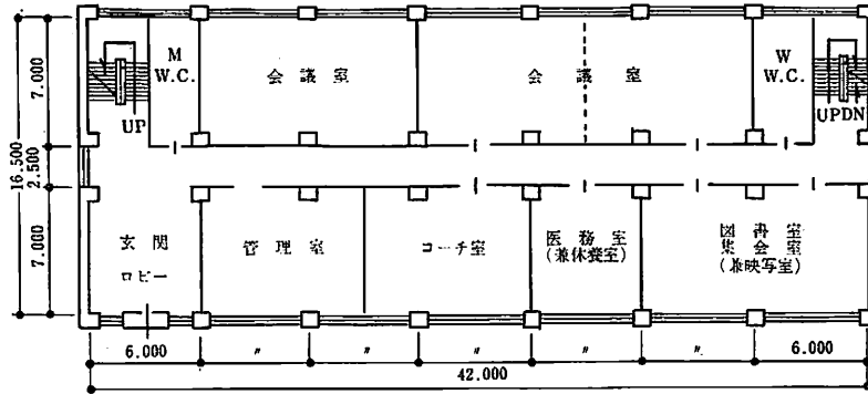
<1階平面図 S:1/300>
